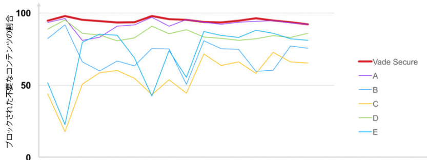
Vade Secureによる脅威のキャッチ率とフィンガープリントベースのソリューションによる脅威のキャッチ率
